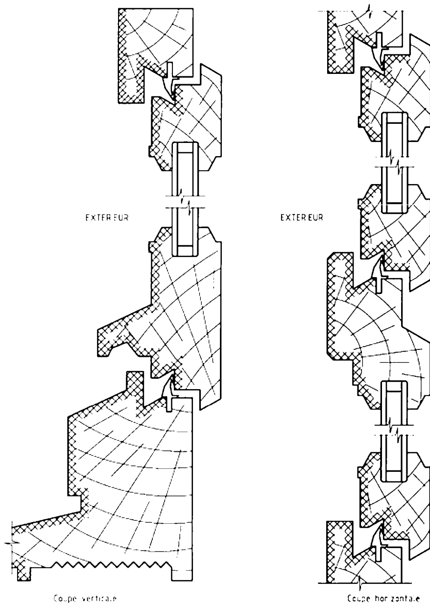
Figure C.2 Fenêtre bois avec joint thermique isophonique
