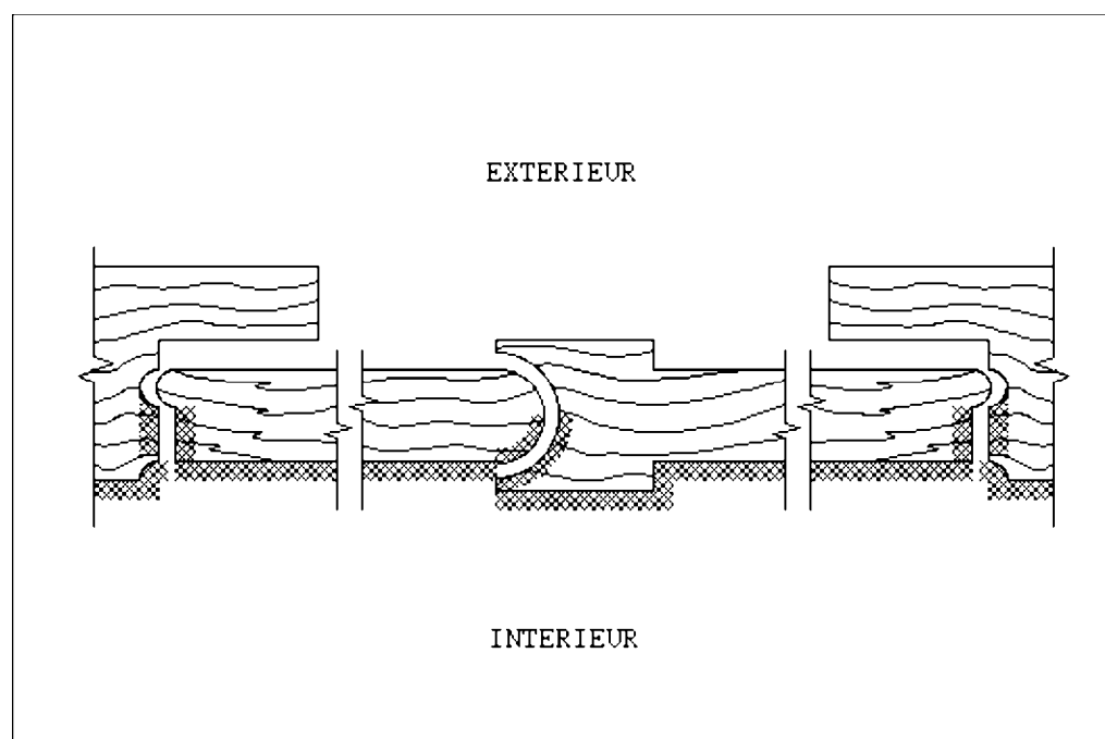
Figure C.1 a) Cas d'une fenêtre bois
