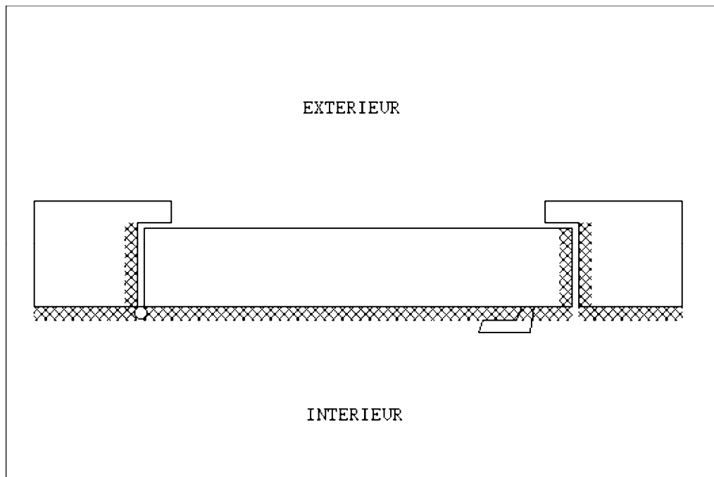
Figure C.1 b) Cas d'une porte à chant plat
