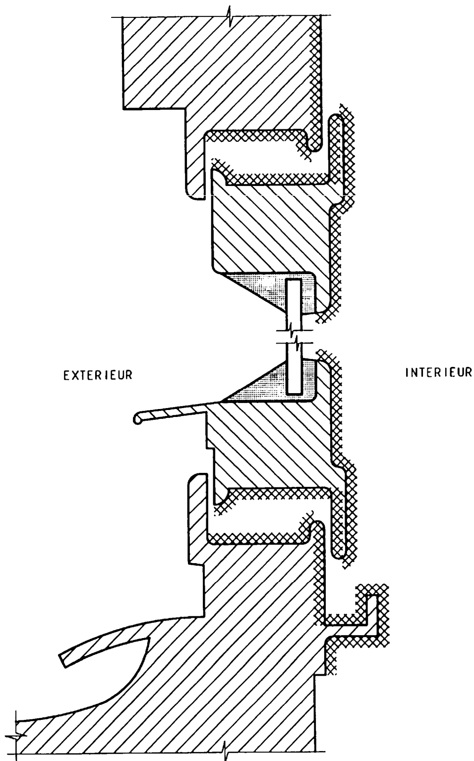
Figure C.3 Cas d'une fenêtre métallique
